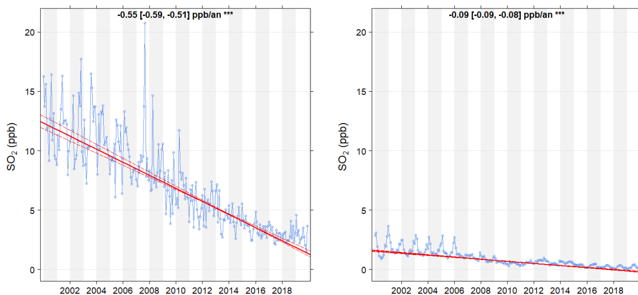
Figure 3.12 Tendence des moyennes mensuelles de dioxyde de soufre à 4 stations industrielles (a) et à 4 stations urbaines (b) pour la période de 2000 à 2019 (20 ans)
