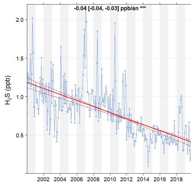
Figure 3.35 Tendance des moyennes mensuelles de sulfure d'hydrogène à la station Trois-Rivières – Cap-de-la-Madeleine pour la période de 2000 à 2019 (20 ans)
